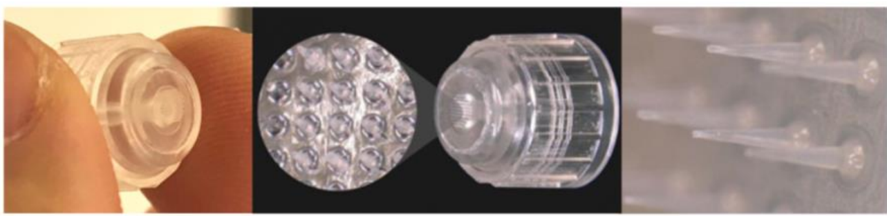
写真左・中央:中空型マイクロニードル 写真右:中空型マイクロニードル先端、貫通孔部分の拡大写真
